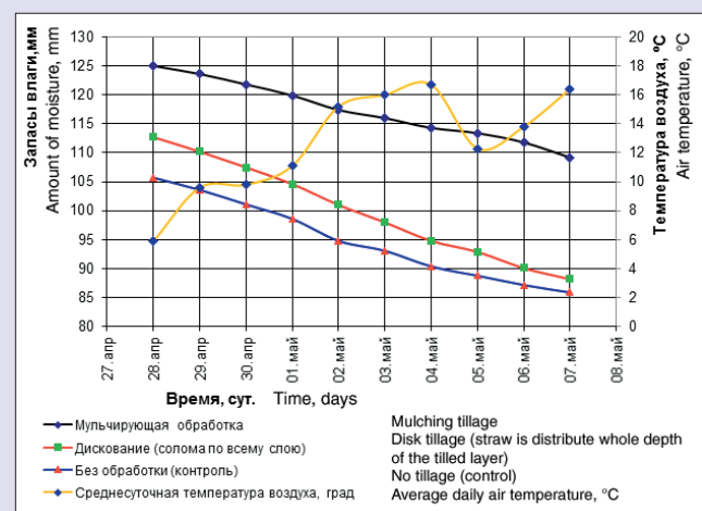
Рис. Изменение общих запасов влаги в пахотном слое в зависимости от видов обработки и среднесуточной температуры воздуха
